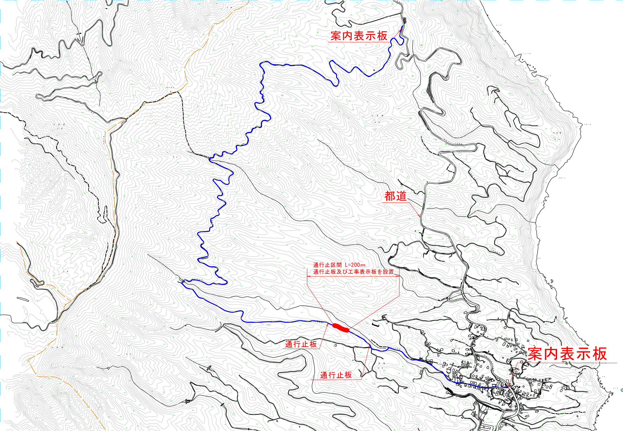
ねぎばな水壺線道路改良工事位置図（看板等配置図）
